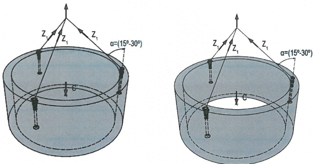
Rysunek 3. Schemat podnoszenia dennic, kręgów przy zawiesiach 3-ciężnowych – równomierny rozkład sił na każdą z kotew
