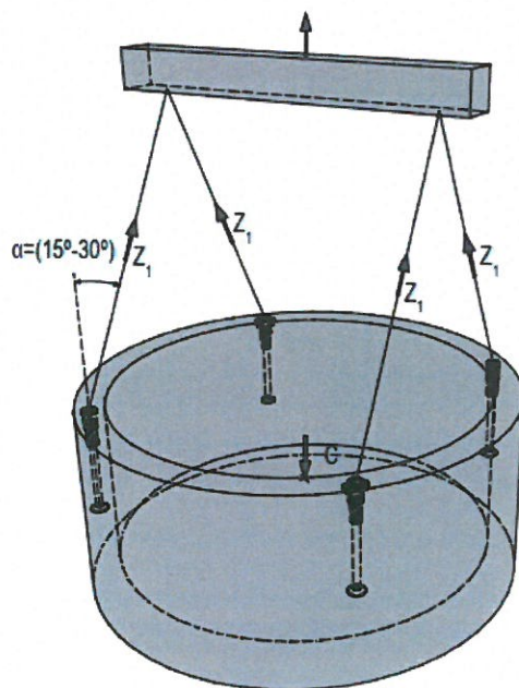
Rysunek 4. Schemat podnoszenia dennic przy zawiesiach 4-ciężnowych z wykorzystaniem belki trawersowej - równomierny rozkład sił na każdą z kotew
